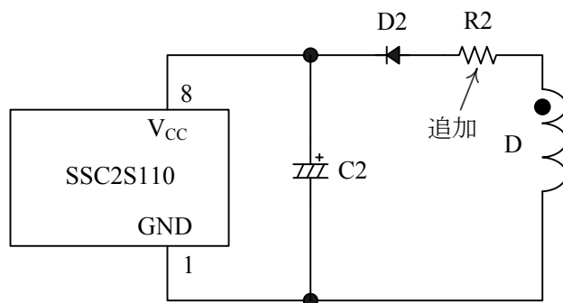
图 7-5 不易受输出电流 I_{OUT} 影响的 V_{CC} 端子周边电路
