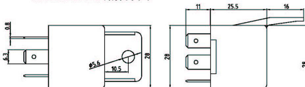
Outline Dimension 外形尺寸 (mm)
